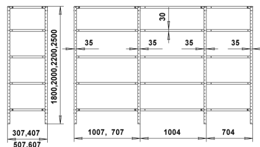
Схема вариантов установки стеллажа СТ-012 ESD
