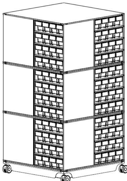
Поворотная кассетница КП-02: 1xКассетница поворотная (без кассет) + 12xКассета К-01/2
