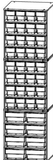
Стационарная кассетница: 1xКассета К-01/1 + 2xКассета К-01/2 + 2xПолка укор. К-01/ПУ ESD
