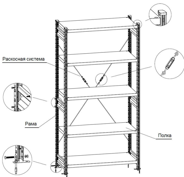
Схема вариантов установки стеллажа СТ-031
