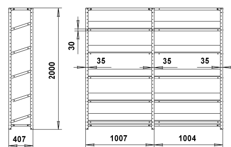
Схема вариантов установки СТ-012 Стеллаж наклонный
