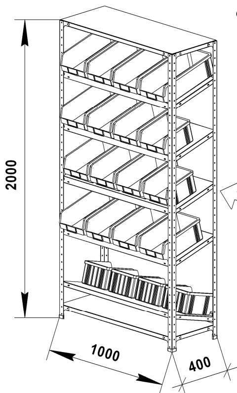
СТ-012 Стеллаж наклонный ESD (без ящиков) 7 310 руб.
